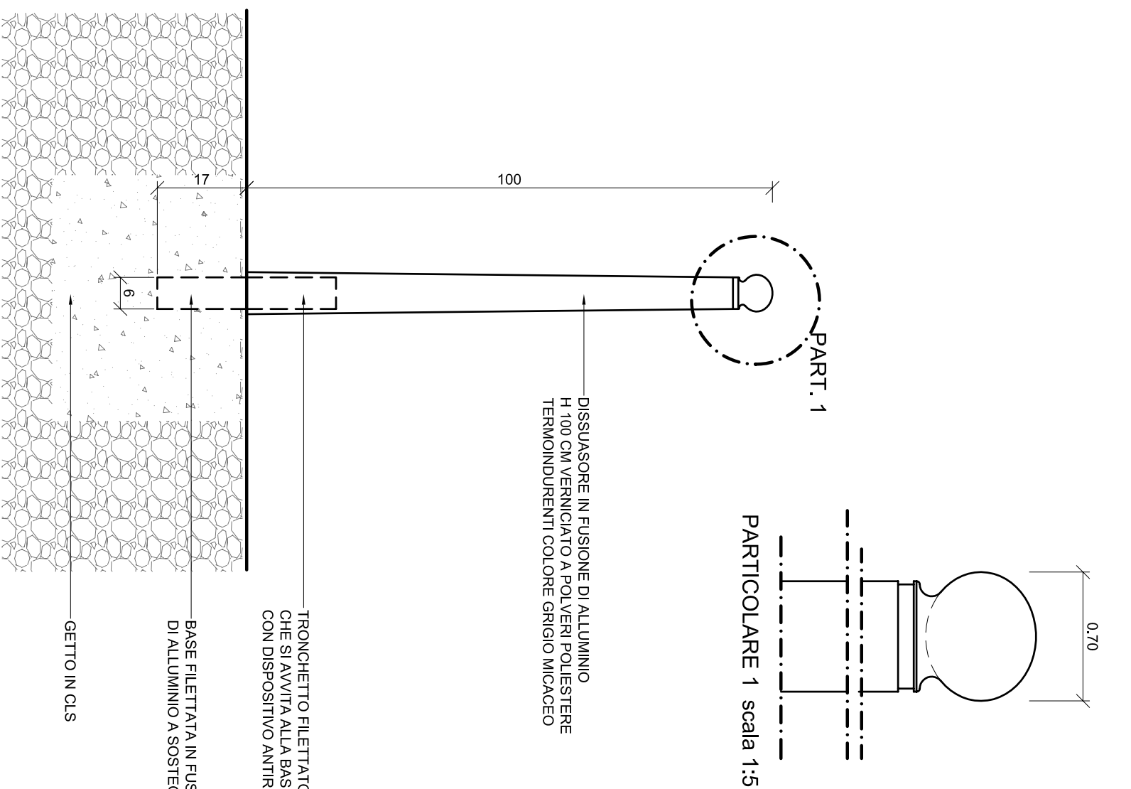
PROSPETTO DISSUASORE scala 1:10
